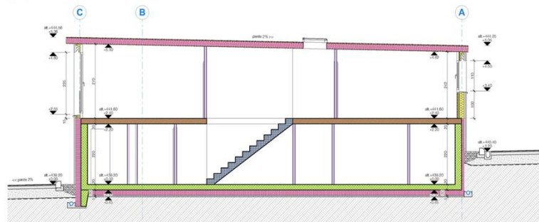
COUPE A-A 1/50
